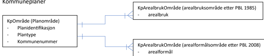
Figur : Datamodell for kommuneplaner
