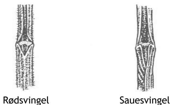
Figur 1. Bladslira hos rødsvingel er sammenvokst (lukka) helt opp til bladkragen, men hos sauesvingel (og stivsvingel) er den øvre delen av bladslira overlappende og åpen. Skillet er mest markert på unge skudd (Stace et al. 1992, Watsonia 19, 107-112)
